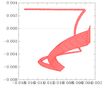
(d) SpaceEx.
