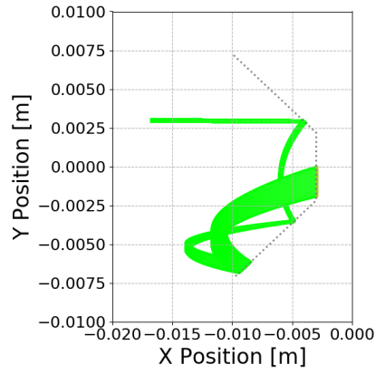
(c) Hylaa.
