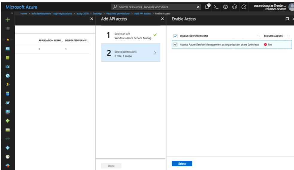
Fig. 6.49: Specifying API permissions
