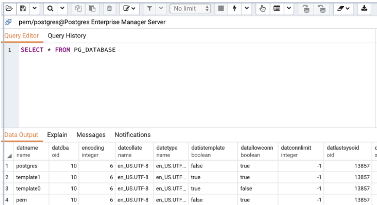
Fig. 2.1: The PEM Query Tool
