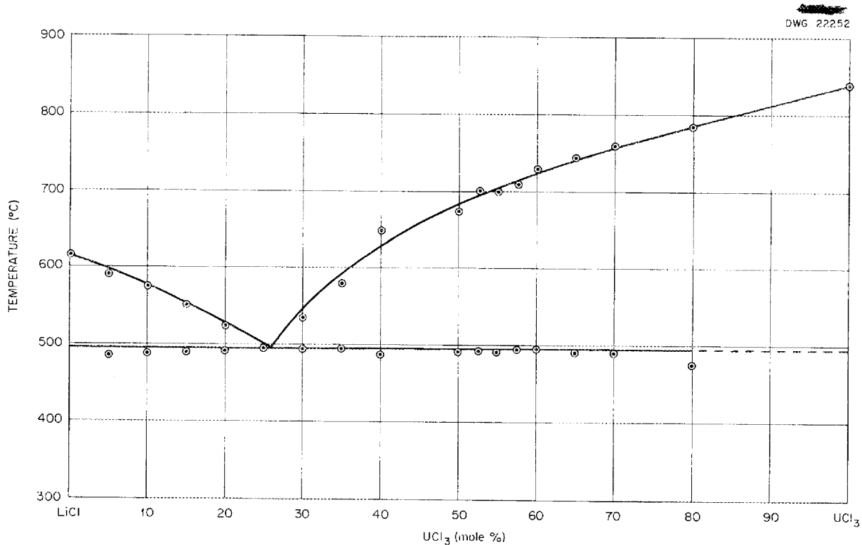
Fig. 5.2. The System LiCl-UCl 3 .
