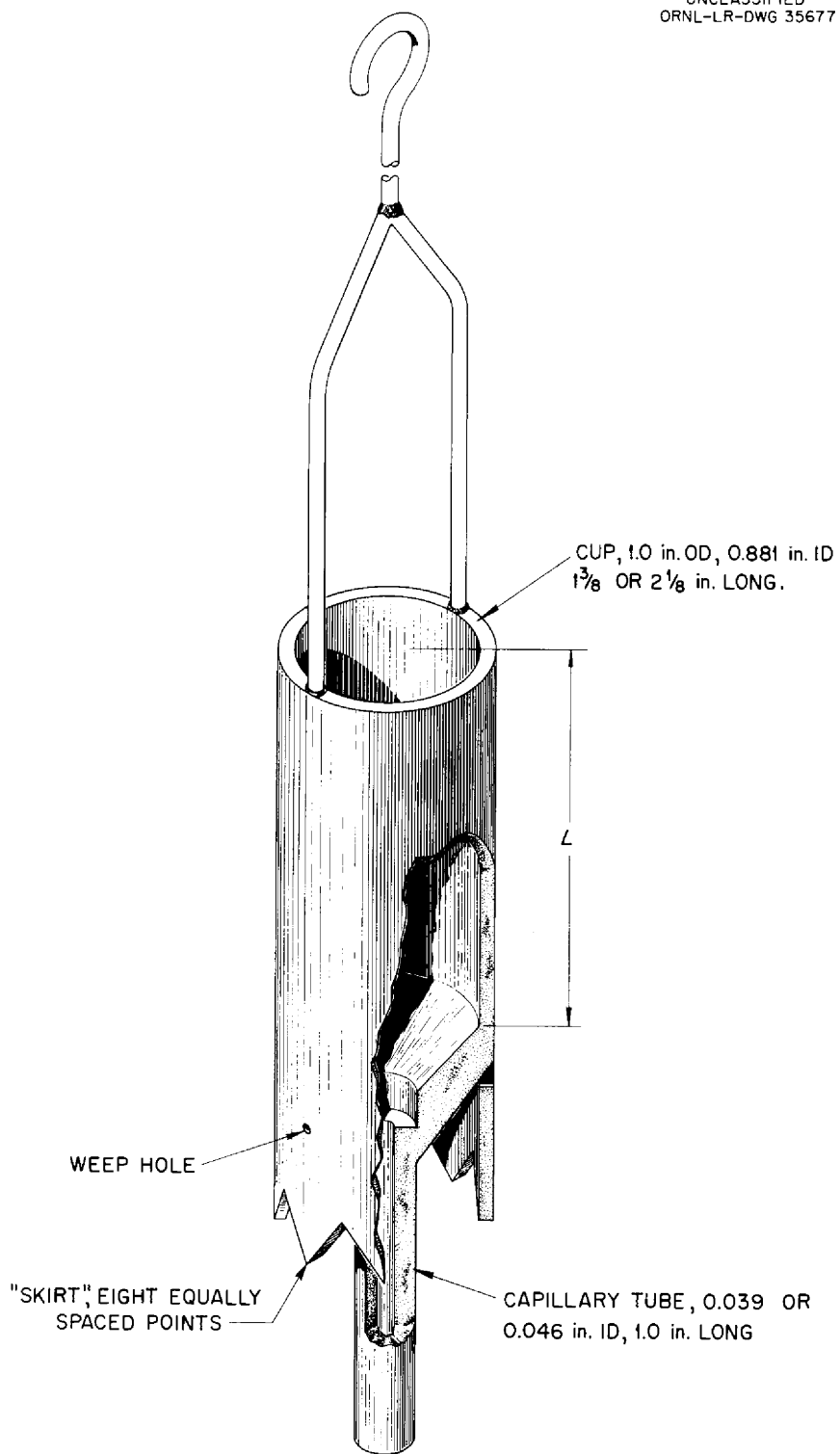
Fig. 1.3.1. Modified Efflux Cup Viscometer.
